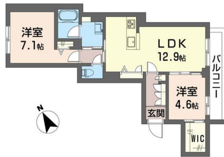
【完成予想図】実際の仕様、色等とは異なる場合がございます。結露中の結露、外灯等はイメージです。
