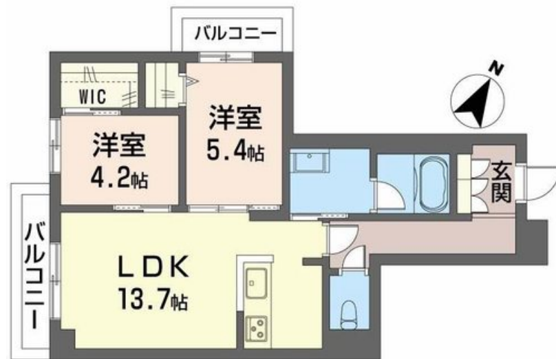
完成予想図
